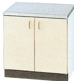
コンロ台 W600×D550×H620mm
