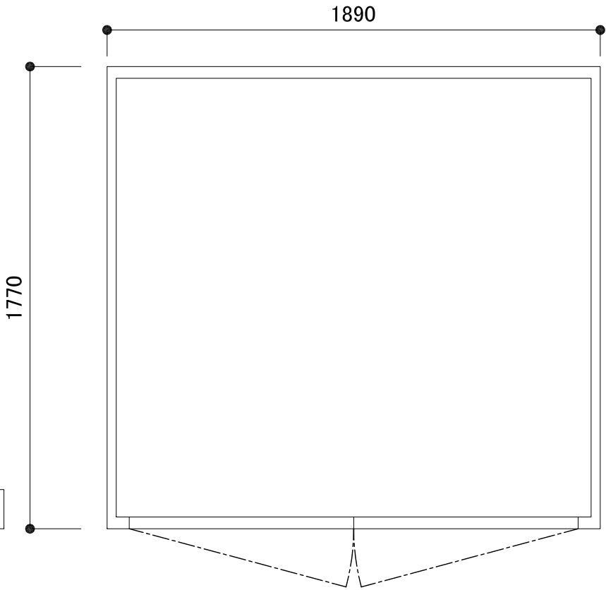
平面図
