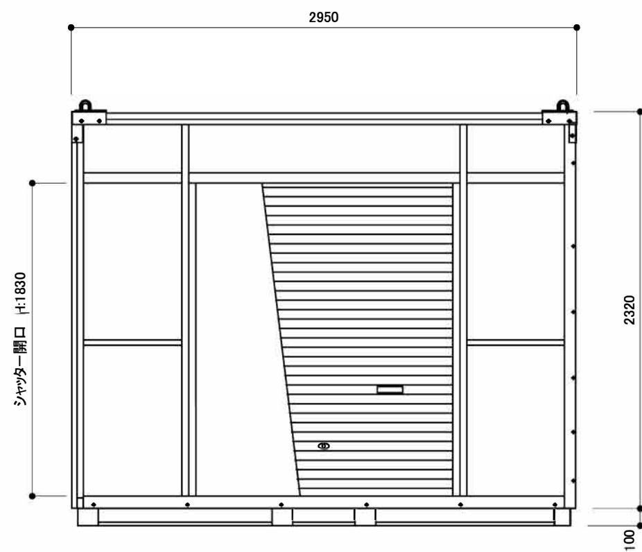
Y通り立面図
