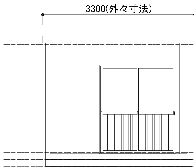
立面図
