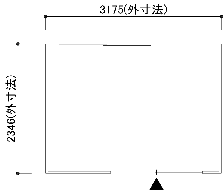
平面図
